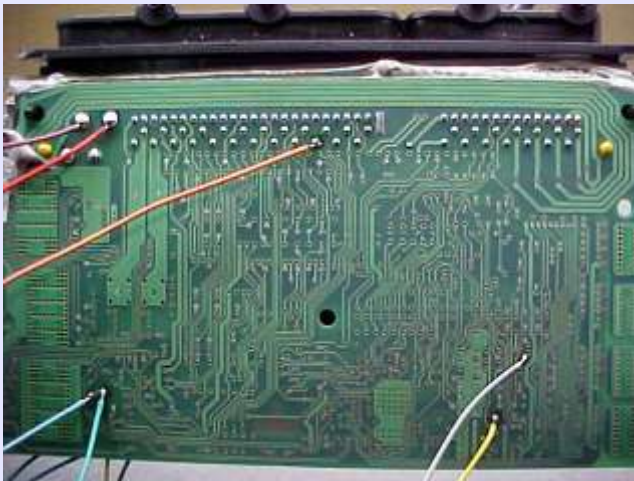
Visualização dos fios cinza e amarelo soldados na Placa de Circuito da Central Magneti Marelli IAW 4SF
