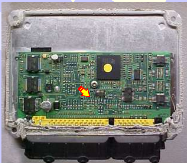
Modo correto de terminar de abrir a Central Magneti Marelli IAW 4DF
