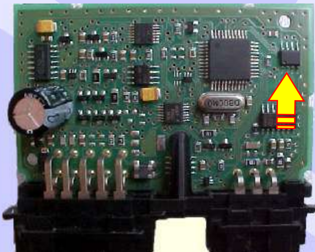
Identificando o pino um da memória (SMD 24C04) do immobilizador..
