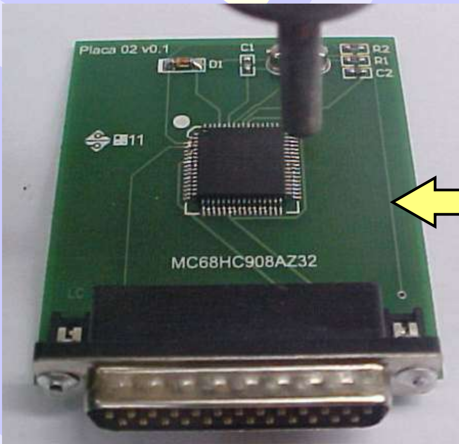
Soldando o processador na placa 02
