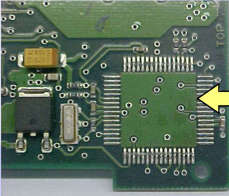
Ilustração mais ampliada da placa de circuito do Imobilizador GM OPEL 2R sem processador
