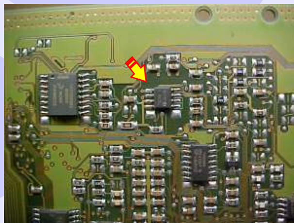
Visualizando a placa de circuito da Central Bosch Motronic ME 7.5.20
